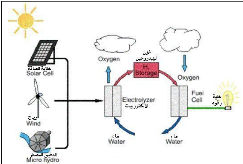
شكل (١١-٤): مخطط يوضح استخدام الهيدروجين لنقل الكهرباء بدلاً من الشبكة الكهربائية.
