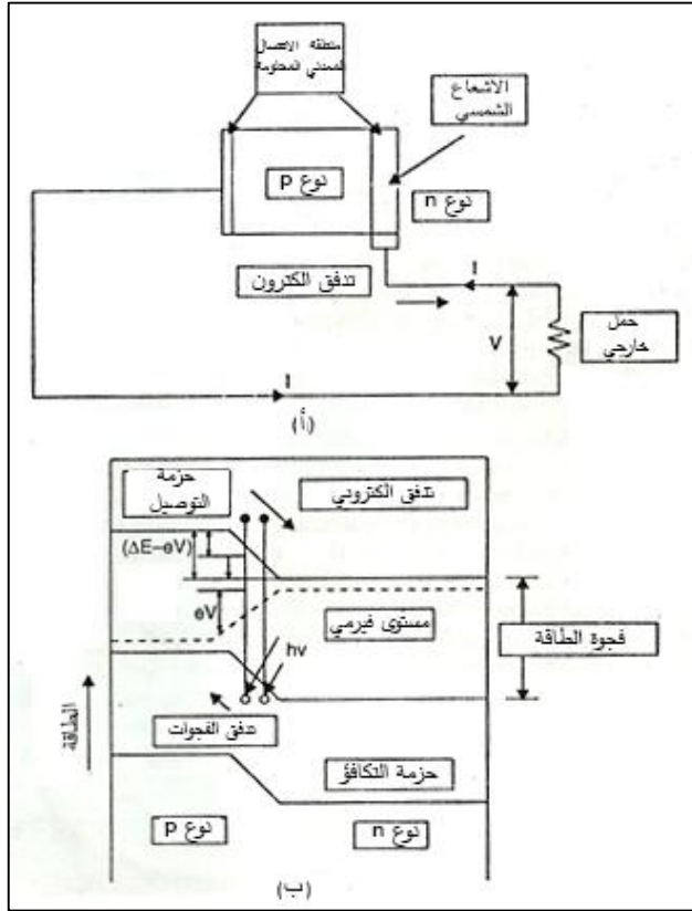
الشكل (3-3): يمثل تشغيل وصلة خلية ضوئية (أ) مخطط وصلة (P-n) (ب)-مخطط مستوى الطاقة.
