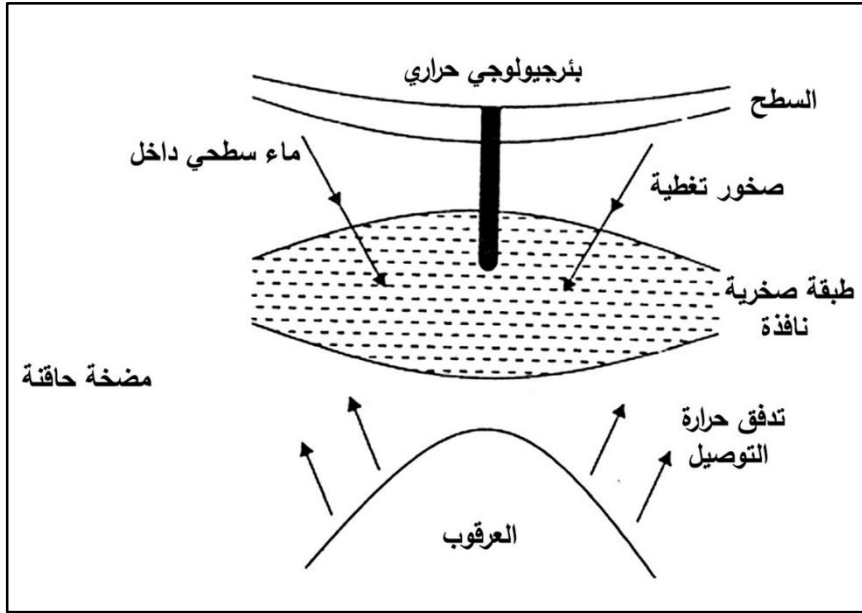
شكل (٨-٥): يوضح نظام الحمل بواسطة الحرارة المائية.
