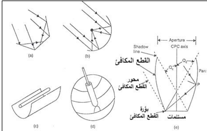
شكل رقم(٤-١٢):الجامعات المركزة (a) صفيحة مستوية وعاكس مستوي (b) قطع مكافئ (c) اسطوانة قطع مكافئ (d) قطع مكافئ (e) اجزاء المركز ذو القطع المكافئ جزء (b) من الشكل يظهر المراكز ذات القطع المكافئ.
