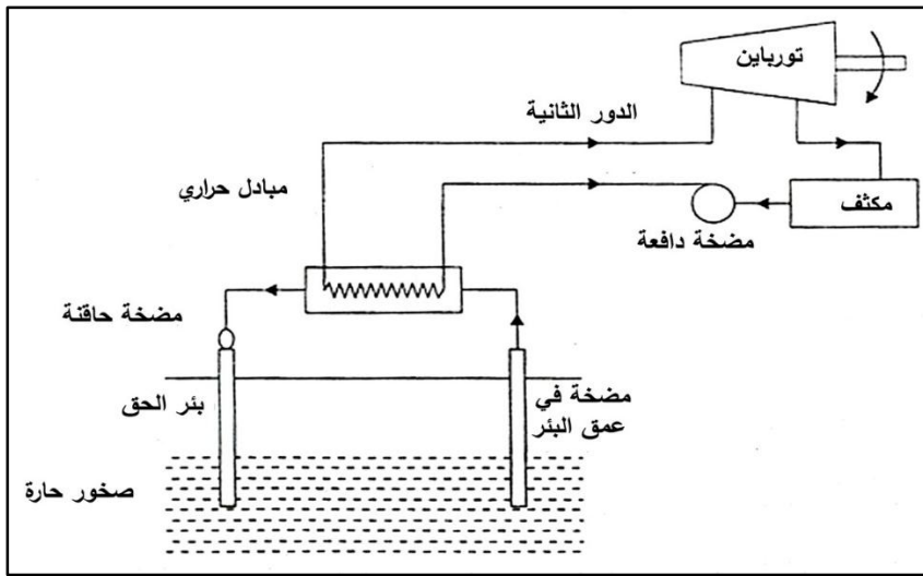
شكل (٢-٨): يبين مخطط لمحطة طاقة حرارة جوفية.
