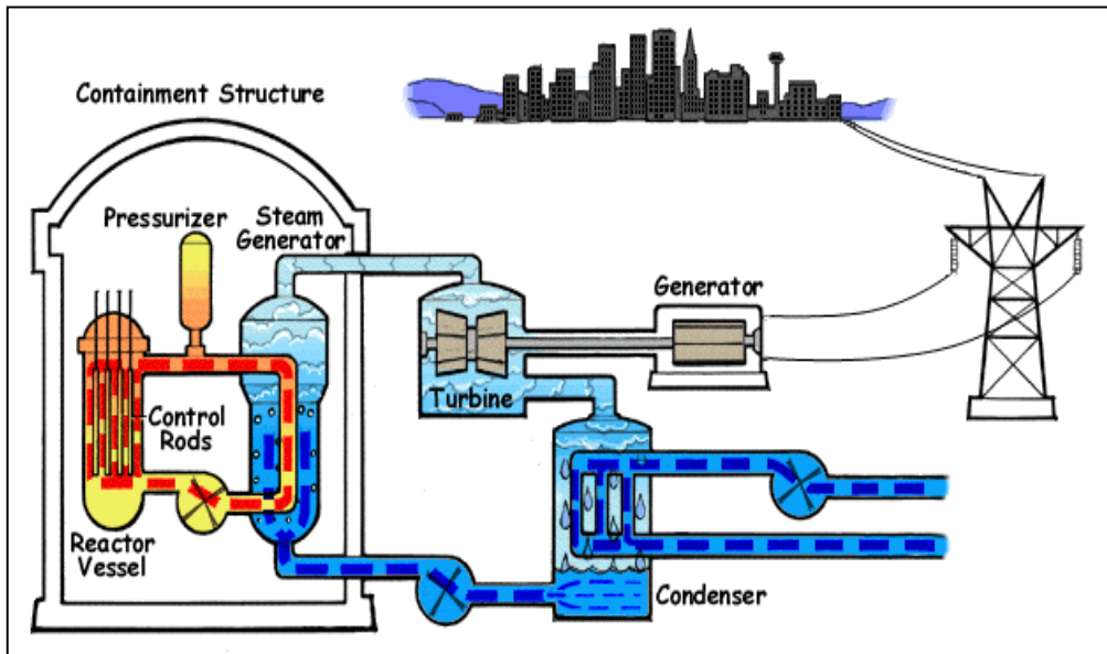
شكل (١٣-٢ ج): يمثل محطة نووية لتوليد الطاقة الكهربائية.
