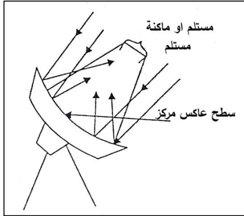
شكل (٤-٢٥): الصحن ذو شكل قطع مكافئ.
