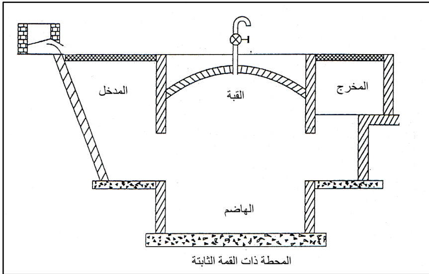
شكل (١٣-٦): يمثل المحطة ذات القبة الثابتة
