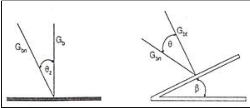
الشكل (٤-٩): يوضح زاوية السقوط للاشعة على سطح افقية وعمودية.
