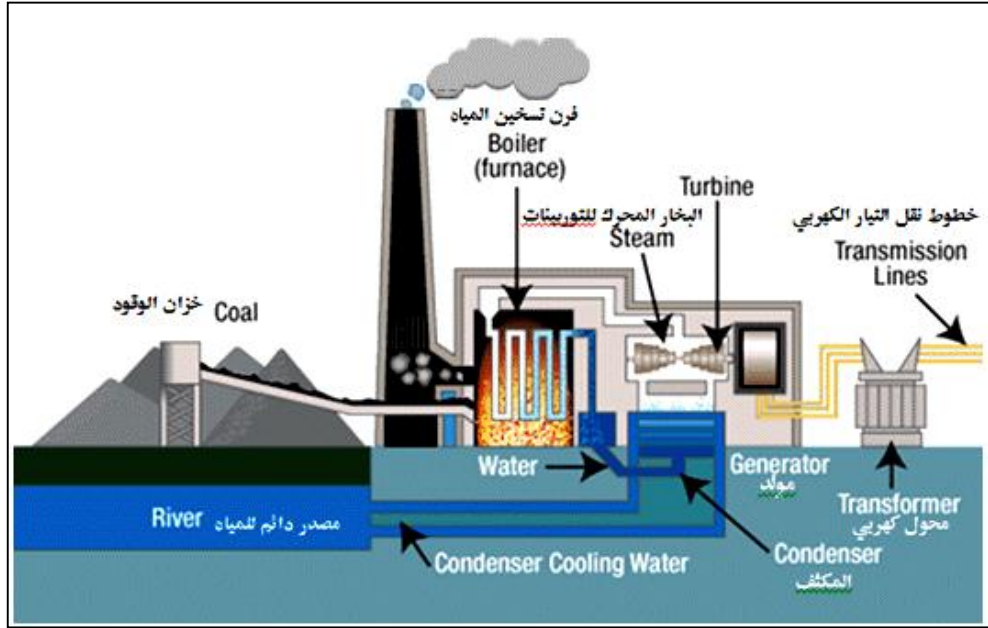
شكل (١٣-٢ ب): يمثل مكونات المحطات البخارية لتوليد الطاقة الكهربائية.
