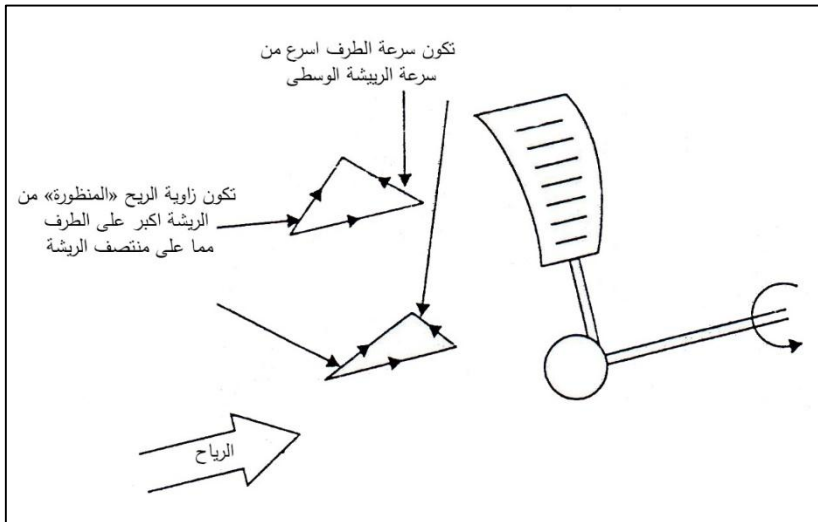
الشكل (٥-٥): تغير زاوية خطران الريش مع نصف القطر.
