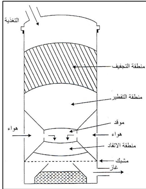
شكل (٦-٧): يمثل محطة السحب الى الاسفل (Downdraft or current gasifier)
