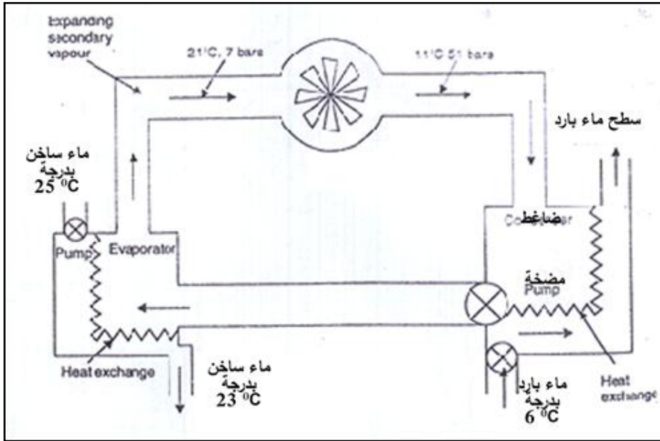
شكل (٩-٣): يمثل نموذج لمحطة تعمل بالدائرة المغلقة لتحويل الطاقة الحرارية لمياه البحار والمحيطات.
