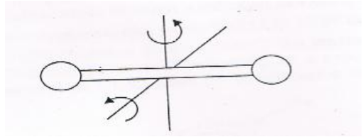
الشكل (١٠-٢): دوار صلب متنقل له درجات دوارنية حرة.
