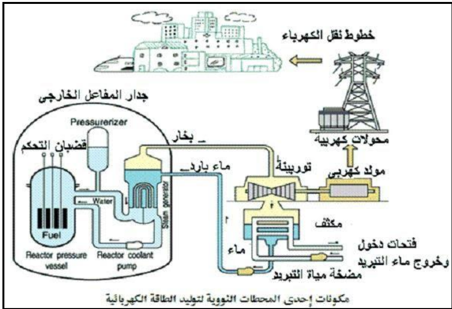
شكل (٢-٣): مكونات إحدى المحطات النووية لتوليد الطاقة الكهربائية.
