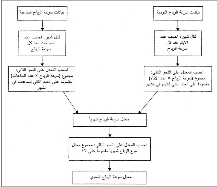
الشكل (١١-٥): مخطط سير العمليات يحدد الخطوات التي يجب اتخاذها عند معالجة بيانات الرياح.
