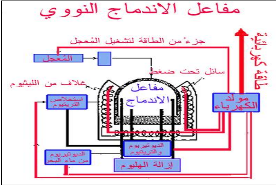
شكل (١٣-١ ج): يمثل مفاعل الاندماج النووي.
