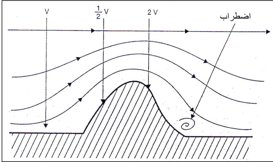
الشكل (٥-١٠): رسم تخطيطي يظهر عوامل تعجيل الرياح التقريبي فوق تلٍ ما.
