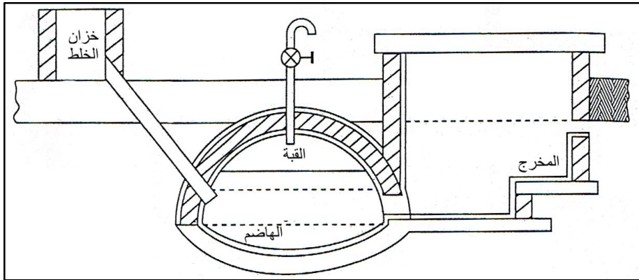
شكل (٦-١٥): يمثل محطة دي باندي موديل.
