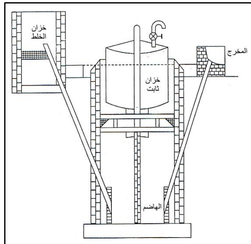
شكل (٦-١٢): يمثل منظومة المحطة العائمة
