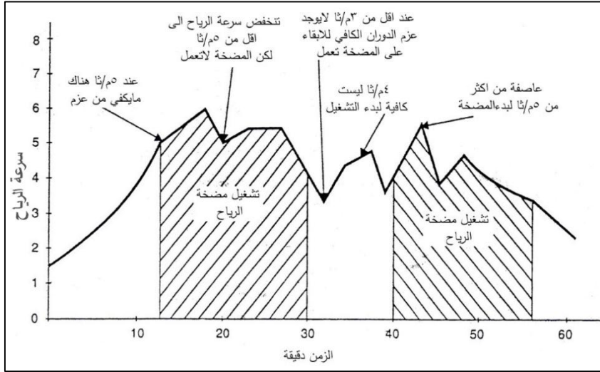
الشكل (٥-٨): يمثل تغير سرعة الرياح مع الزمن.
