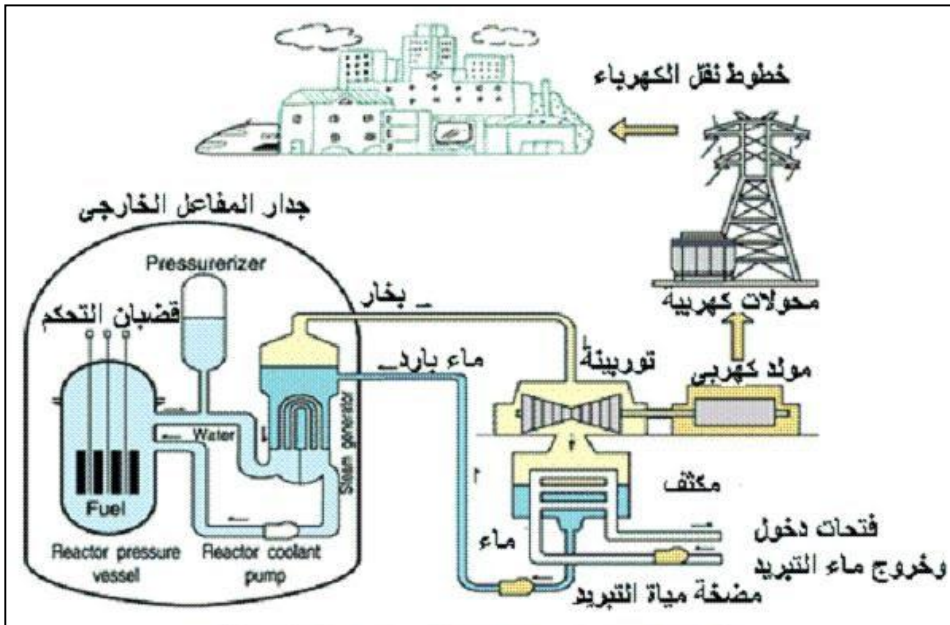
شكل (١٣-٢ أ): يمثل مكونات المحطات النووية لتوليد الطاقة الكهربائية.
