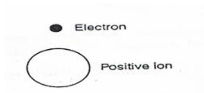
الشكل (١٠-٥): تأين الذرة.
