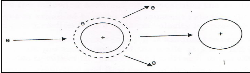
الشكل (١٠-٦): التصادم الأيوني للالكترون.
