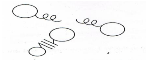
شكل (١٠-٤): انفصال جزيئه الى ذرات متعادلة.
