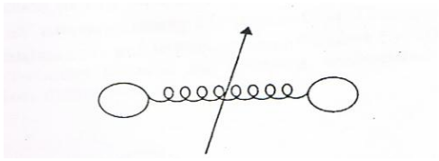
الشكل (١٠-٣) جزيئه ثنائية لها انتقالية دوارنية ودرجات اهتزازية حرة.
