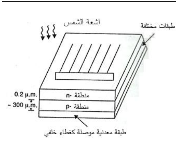
الشكل (٣-٥): مخطط الترتيب الفيزيائي لخلية شمسية نمطية.
