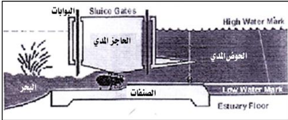
شكل (٩-١): يمثّل المكونات الرئيسية لمحطة المد والجزر.
